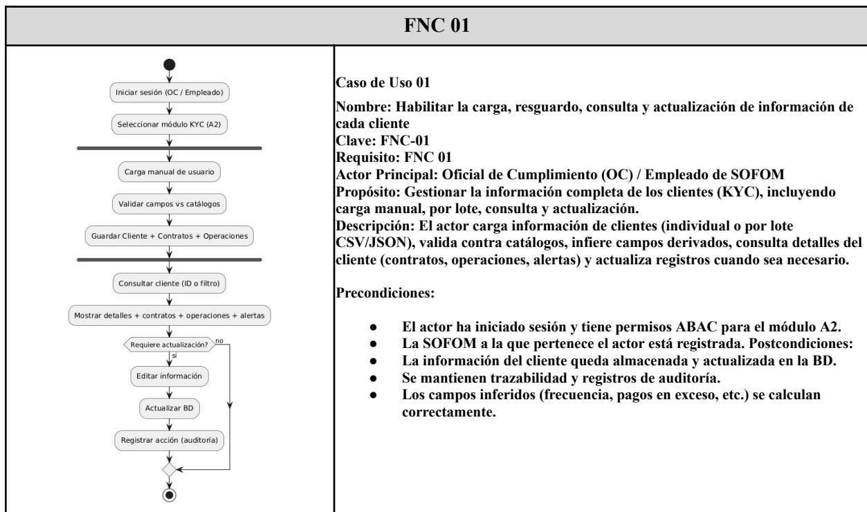
Figura 2. Detalles del Caso de Uso 01 y Diagrama de Actividades
