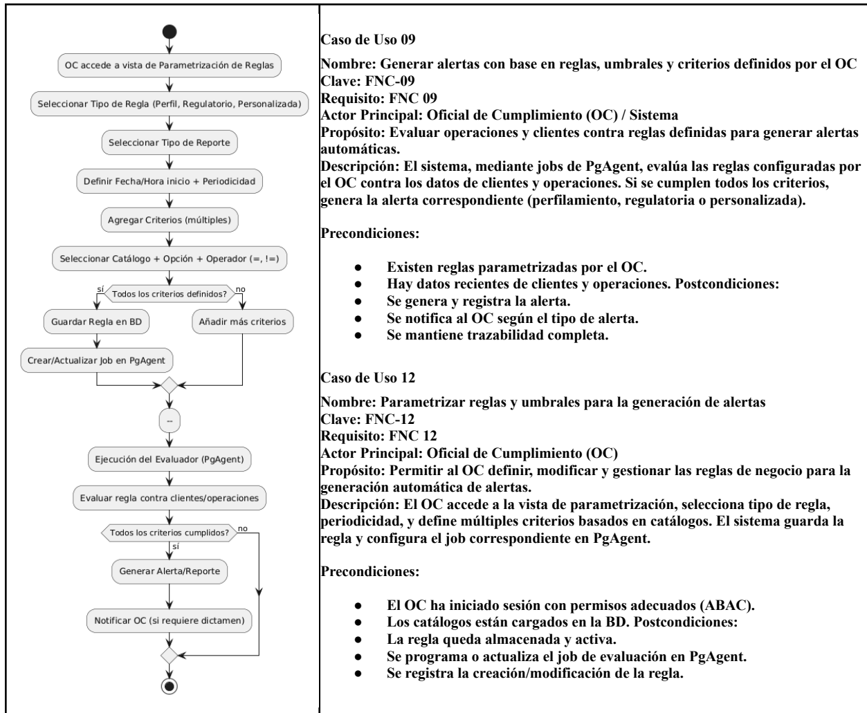
Figura 4. Detalles del Caso de Uso 09/12 y Diagrama de Actividades
