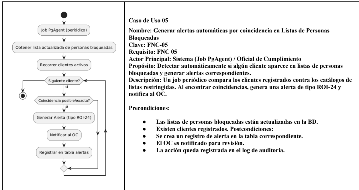
Figura 3. Detalles del Caso de Uso 05 y Diagrama de Actividades
