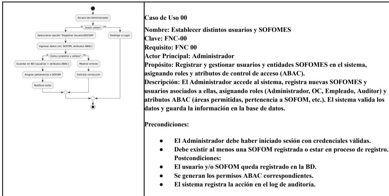
Figura 1. Detalles del Caso de Uso 00 y Diagrama de Actividades.
