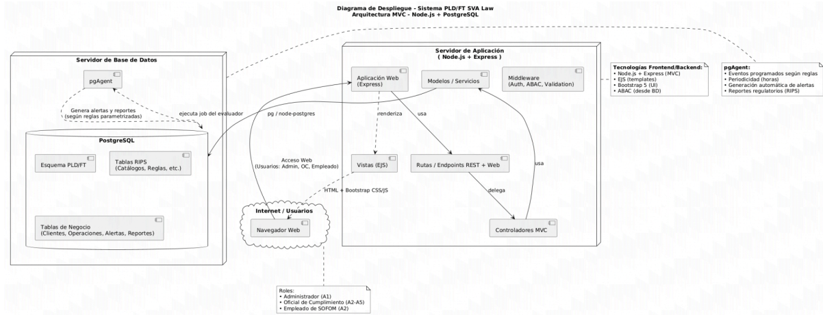
Figura 7 - Diagrama de despliegue entre los distintos actores y componentes del sistema
