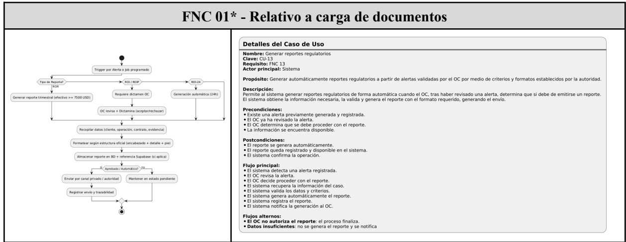
Figura 6. Detalles del Caso de Uso 13 y Diagrama de Actividades
