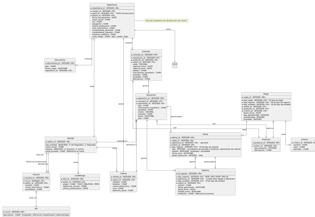
Figura 7 - Modelo Entidad-Relación para Sistema Automático SVA Law. [Diccionario de información]
